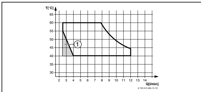
12 ábra +15 °C befolyó hidegvíz hőmérséklet diagramm (ZWC 24-3 MFA/MFK)
